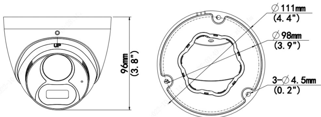
HAC-T325-F28(40)M-W
